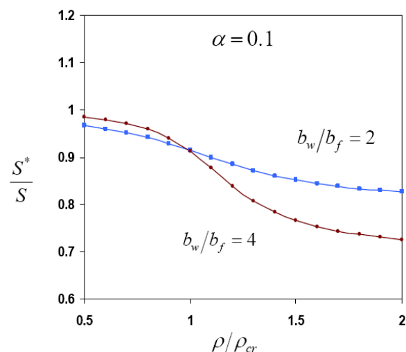
شکل ۵- تغییرات سختی مؤثر بر حسب تغییرات انحناى مقطع Z شکل تحت خمش خالص حول محور ضعیف
