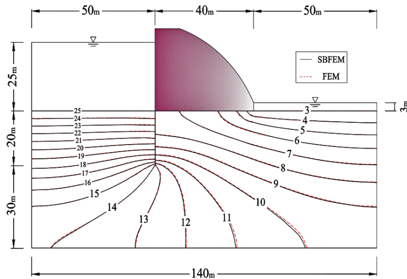
شکل ۱۷- مقایسه خطوط هم پتانسیل جریان حاصل از FEM و SBFEM
