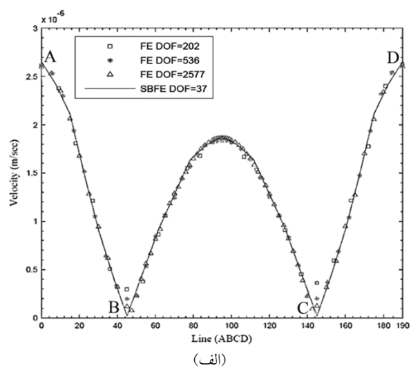
شکل ۱۲- مقایسه مقادیر سرعت جریان الف) در راستای خط ABCD ب) در راستای خط EFG
