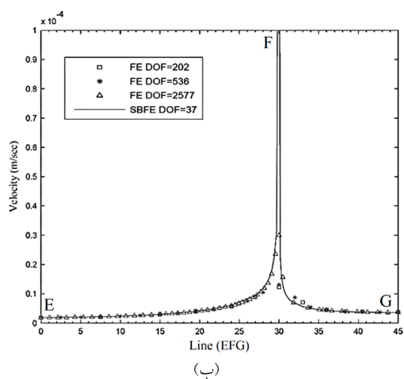
شکل ۱۲- مقایسه مقادیر سرعت جریان الف) در راستای خط ABCD ب) در راستای خط EFG
