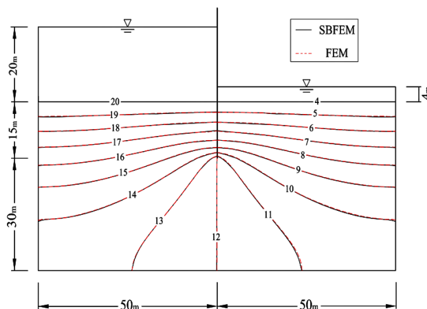
شکل ۱۳- مقایسه خطوط هم پتانسیل حاصل از FEM و SBFEM
