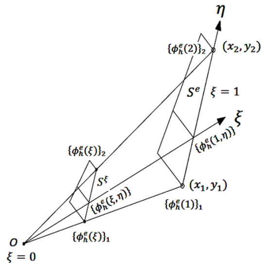
شکل ۳- درونیابی همد داخل حوزه با استفاده از توابع هد گره‌ای
