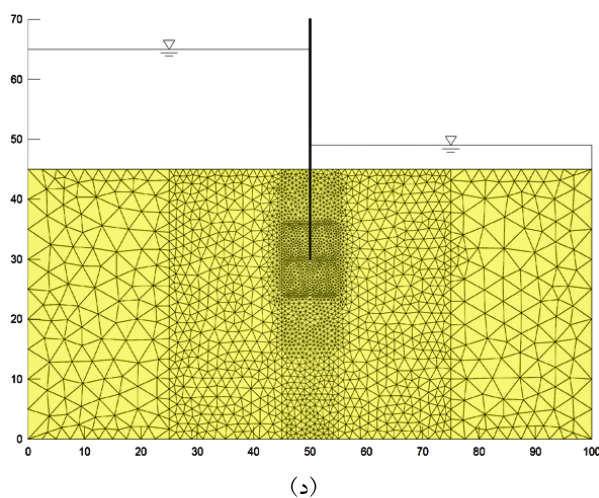
شکل ۱۱- مدل سازی جریان آب در زیر یک ردیف سپری با روشهای اجزای محدود با مرز مقیاس شده و اجزای محدود: الف) SBFEM با ۳۷ درجه آزادی، ب) FEM با ۲۰۲ درجه آزادی، ج) FEM با ۵۳۶ درجه آزادی، د) FEM با ۲۵۷۷ درجه آزادی
