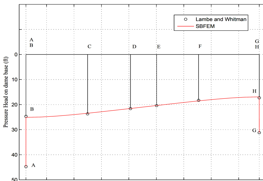
شکل ۸- مقایسه مقادیر هد فشار در زیر سد و نوک سپری
