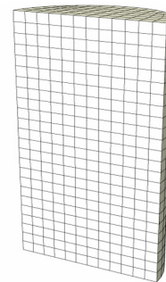
اجزای سه بعدی ۸ گره‌ای C3D8R مورد استفاده قرار گرفته در مدل‌های A-1 و B-1
