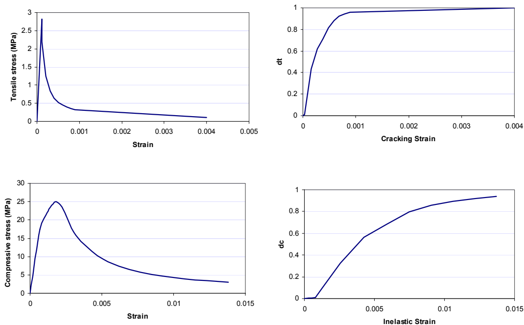
شکل ۳- منحنیهای تنش- کرنش بتن در کشش و فشار و پارامترهای خسارت در کشش و فشار d_t و d_c
