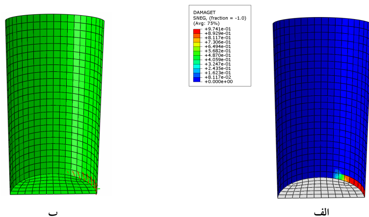
شکل ۵- الف) خسارت در کشش در مدل A-1 ب) جهت بردارهای عمود بر صفحه ترکها در مدل A-1
