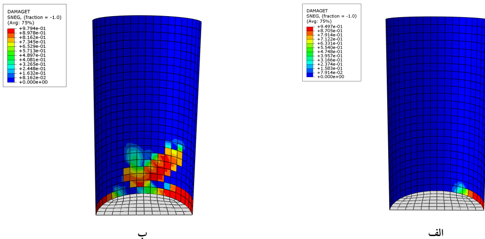
شکل ۱۶- الف) خسارت در کشش در مدل B-1 با فرض n = 0/28 ب) خسارت در کشش در مدل B-1 با فرض n = 0/39
