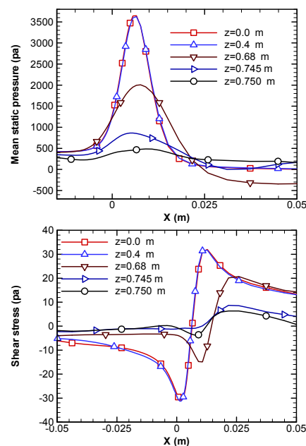
شکل ۱۳- توزیع فشار و تنش برشی در موقعیتهای مختلف در عرض ورق در حالت اول
