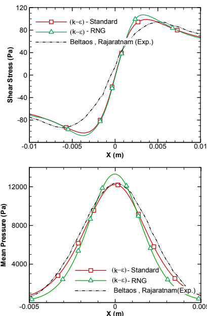
شکل ۴- مقایسه توزیع فشار و تنش برشی در طول ورق با مدل های مختلف توربولانس
