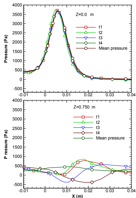
شکل ۱۴- توزیع فشار در طول ورق در زمانهای مختلف، بالا: در مرکز ورق، پایین: در لبه ورق
