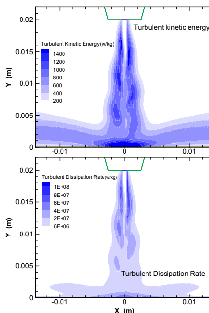
شکل ۸- کانتورهای انرژی جنبشی و نرخ استهلاک توربولانس
