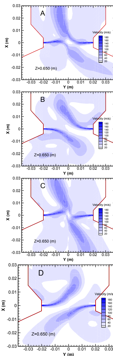
شکل ۱۸- کانتورهای سرعت ناش از برخورد دو جت در فاصله 25 mm بعد از لبه ورق در زمانهای مختلف در حالت دوم
