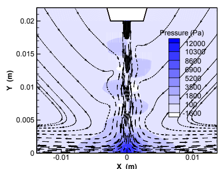
شکل ۱۰- خطوط جریان به همراه کانتورهای فشار
