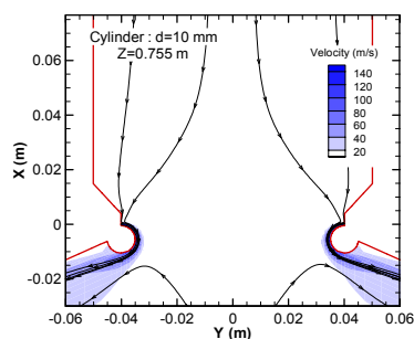
شکل ۲۳- کانتور سرعت و خطوط جریان در موقعیتهای مختلف عرضی ورق در هنگام استفاده از تجهیز استوانه‌ای
