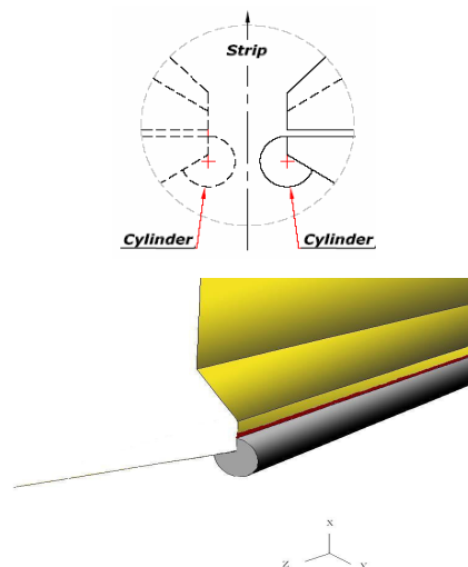
شکل ۲۲- نحوه قرارگیری دو استوانه در دو طرف ورق و زیر لبه پایینی جتها
