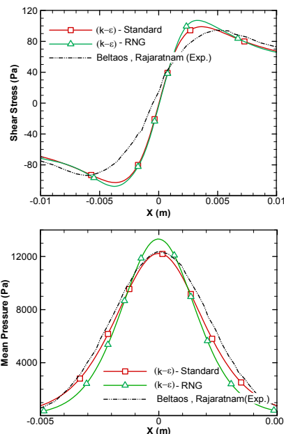
شکل ۴- مقایسه توزیع فشار و تنش برشی در طول ورق با مدل های مختلف توربولانس
