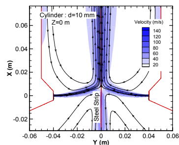
شکل ۲۲- نحوه قرارگیری دو استوانه در دو طرف ورق و زیر لبه پایینی جتها
