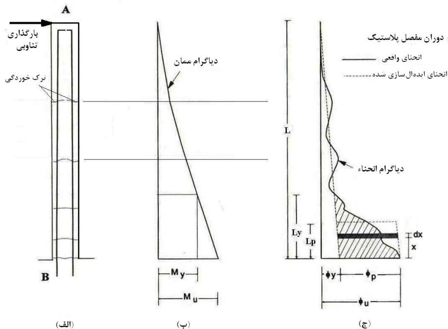
شکل ۲- توزیع نمایشی انحنای در راستای ستون در مرحله بار نهایی؛ (الف) ستون؛ (ب) نمودار گشتاور خمشی؛ (ج) نمودار انحنای
