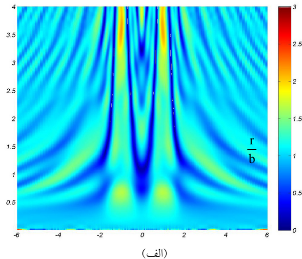
شکل ۴- نمودار بزرگنمایی حرکت افقی تپه‌های با نسبت شکل ۰/۵؛ (الف) تپه‌های مرکب دوگانه همسان، (ب) تپه منفرد. [محورهای افقی و قائم به ترتیب، فاصله از مرکز عارضه توپوگرافی (شکلهای (۱-الف) و (۱-ج)) و فرکانس بدون ( \Omega ) بعد را نمایش می‌دهند].
