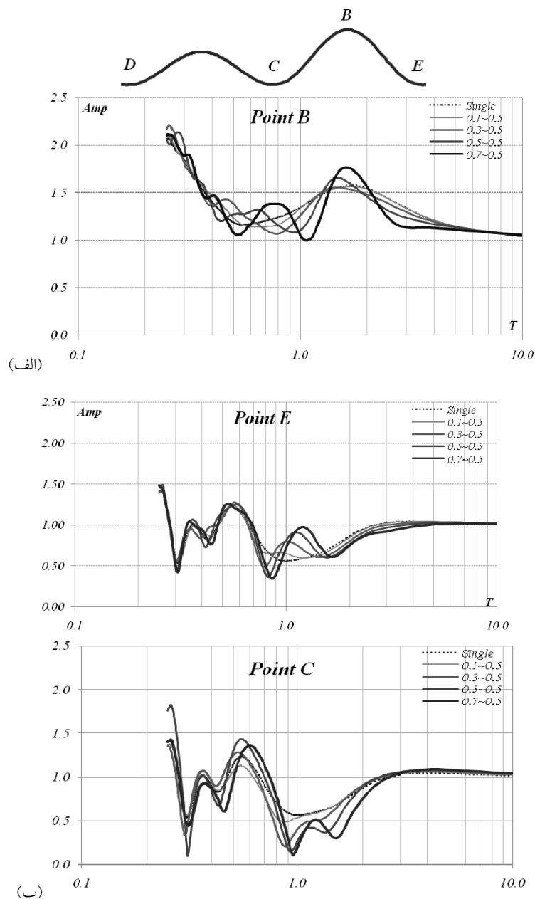
شکل ۸- منحنیهای بزرگنمایی تاج، کناره داخلی و خارجی تپه مرجع با نسبت شکل ۵/۰ در تپه‌های ناهمسان به ازای نسبتهای شکل ۱/۰، ۳/۰، ۵/۰ و ۷/۰ برای تپه مجاور؛ (الف) تاج، (ب) کناره داخلی و خارجی
