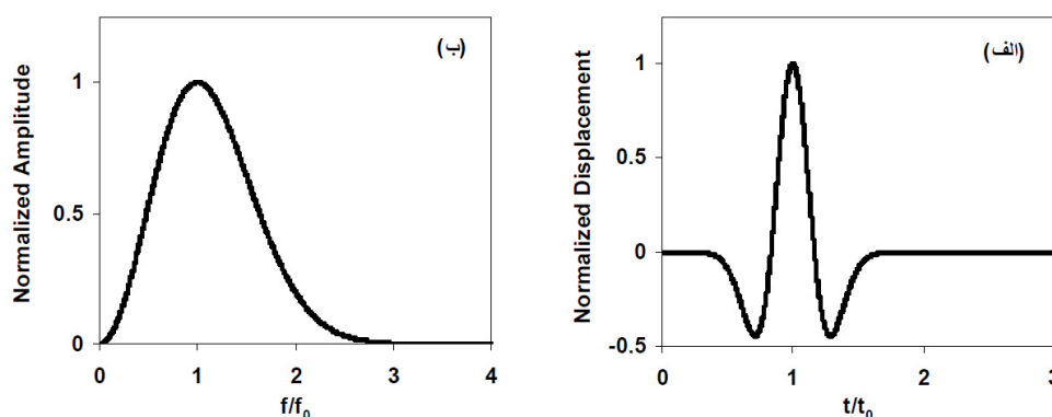
شکل ۳- تاریخچه زمانی و طیف فوریه موج ریکر
