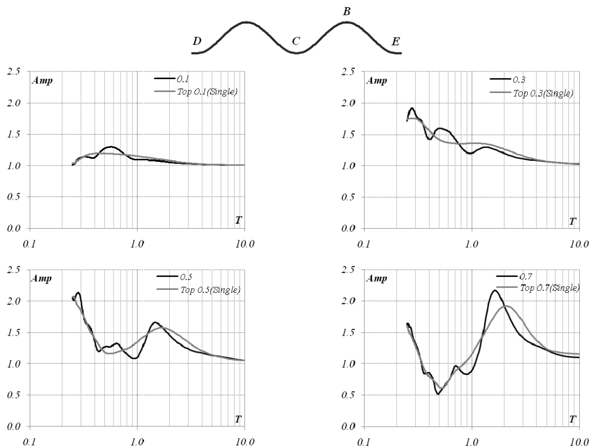
شکل ۵- منحنیهای بزرگنمایی تاج تپه‌های همسان (نقطه B) به ازای نسبت‌های شکل ۰/۷ و ۰/۵، ۰/۳، ۰/۱ [محور افقی، پی‌ریود بدون بعد (T در معادله (۶)) را نمایش می‌دهد].
