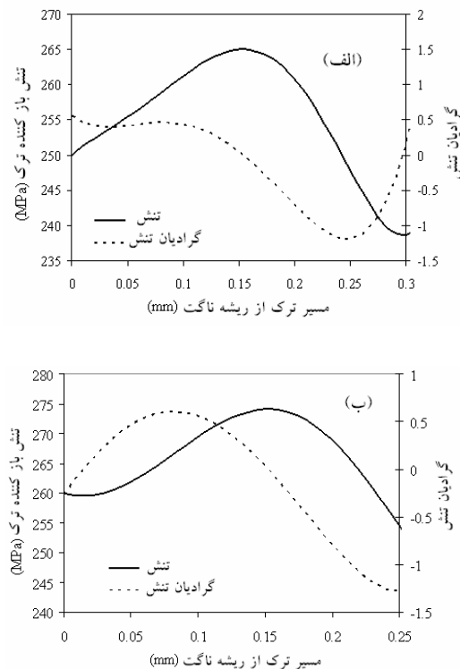
شکل ۸- توزیع تنش الاستیک-پلاستیک و گرادیان نسبی تنش در امتداد مسیر ترک از ریشه ناگت‌ها به ازای بار اعمالی به مقدار ۵۰٪ بار شکست استاتیکی الف) فاصله‌ی بین صفحات ۰/۰۹ میلی‌متر، ب) فاصله‌ی بین صفحات ۰/۱۱ میلی‌متر، ج) فاصله‌ی بین صفحات ۰/۱۳ میلی‌متر
