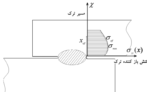
شکل ۳- امتداد تنش باز کننده ترک در برابر مسیر ترک در اتصالات نقطه جوش
