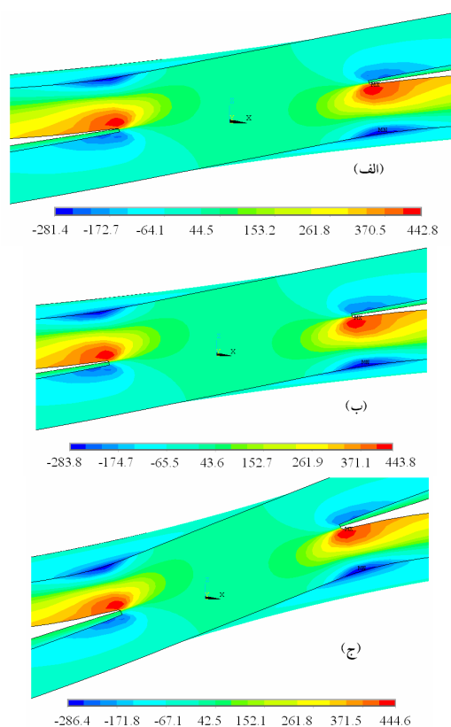
شکل ۹- منحنی تنش در مجاورت ریشه فاق برای بار اعمالی به میزان ۸۰٪ بار شکست استاتیکی برای سه نوع اتصال نقطه جوش (الف) فاصله‌ی صفحه ۰/۰۹ میلی‌متر، (ب) فاصله‌ی صفحه ۰/۱۱ میلی‌متر، (ج) فاصله صفحه ۰/۱۳ میلی‌متر (تنش‌ها بر حسب مگاپاسکال می‌باشد)
