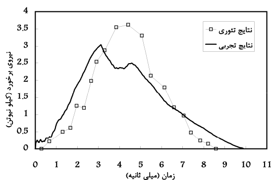
شکل ۵- نیروی برخورد نظری و تجربی برای نمونه نایلون خالص
