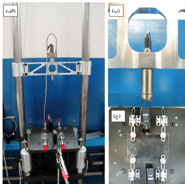
شکل ۴- نمایش از (الف) دستگاه ضربه، (ب) شکل ضربه زن و (ج) نحوه بستن نمونه در دستگاه
