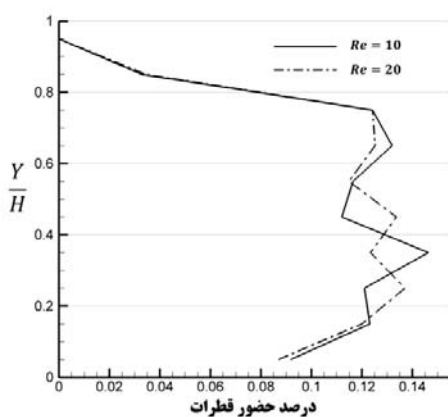
شکل ۶- تأثیر عدد رینولدز برای \gamma=3.0, Ca=0.8, \alpha=30^\circ, \lambda=2.0
