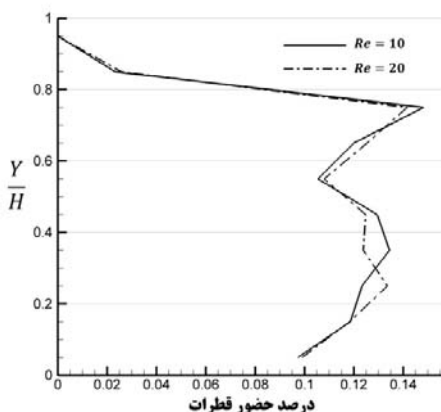
شکل ۴- تأثیر عدد رینولدز برای Ca=0.8, \alpha=10^\circ, \lambda=2.0, \gamma=3.0
