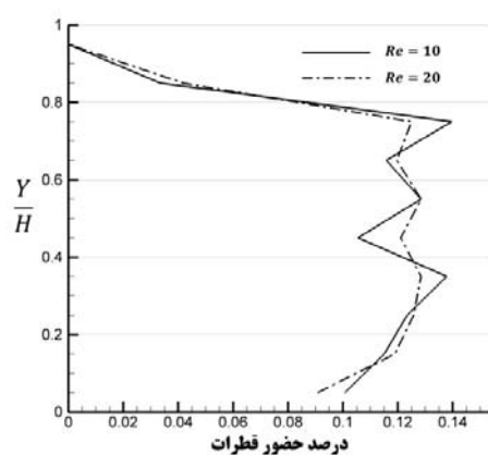
شکل ۷- تأثیر عدد رینولدز برای Ca=0.8, \alpha=30^\circ, \lambda=2.0, \gamma=4.0
