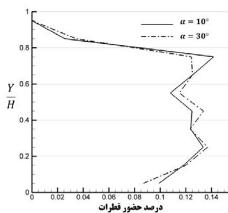
شکل ۱۰- تأثیر زاویه شیب سطح برای Re=20, Ca=0.8, \lambda=2.0, \gamma=3.0
