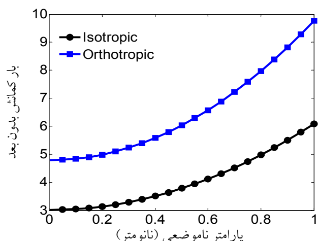
شکل ۱۱- اثر خواص الاستیک بر بار کمانش بدون بعد گرافین به ازای شرایط تکیه گاهی ساده- با اعمال تئوری گرادیان کرنش مرتبه دو
