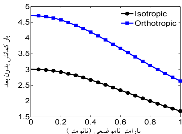
شکل ۱۰- اثر خواص الاستیک بر بار کمانش بدون بعد گرافین به ازای شرایط تکیه گاهی ساده- با اعمال تئوری غیرمحملی کاهیده
