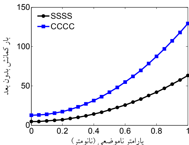
شکل ۹- بار کمانش بدون بعد بر حسب ضریب غیرمحملی برای صفحه گرافین به‌ازای شرایط تکیه‌گاهی ساده و گیردار- با اعمال تئوری زوج تنش تغییر یافته
