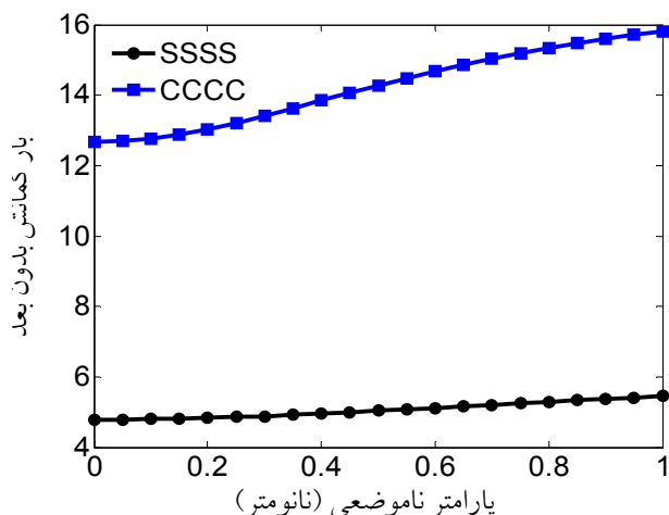
شکل ۸- بار کمانش بدون بعد بر حسب ضریب غیرمحملی برای صفحه گرافین به‌ازای شرایط تکیه‌گاهی ساده و گیردار- با اعمال تئوری گرادیان ضمنی مرتبه دو
