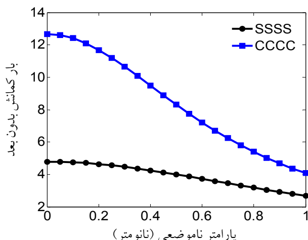
شکل ۶- بار کمانش بدون بعد بر حسب ضریب غیر محلی برای صفحه گرافین به‌ازای شرایط تکیه‌گاهی ساده و گیردار- با اعمال تئوری غیرمحملی کاهیده
