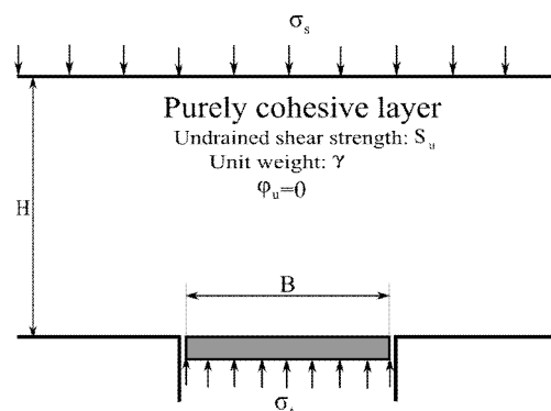
شکل ۷- جزییات مسئله دریچه مدفون
