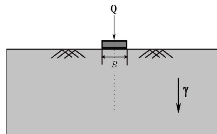
شکل ۶- خاک چسبنده - اصطکاکی با در نظر گرفتن وزن خاک تحت پی نواری
