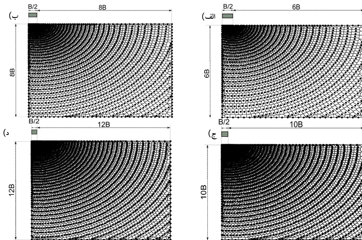
شکل ۵- مدل بدون شبکه برای الف) \phi' = 10^\circ ب) \phi' = 20^\circ ج) \phi' = 30^\circ د) \phi' = 40^\circ
