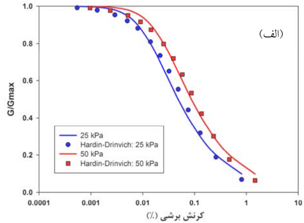
شکل ۱۰- الف) منحنی های G/G_{max} کالیبره شده آزمایشات با مدل هاردین-درینویچ؛ ب) چرخه هیستریزس تنش-گرنش
