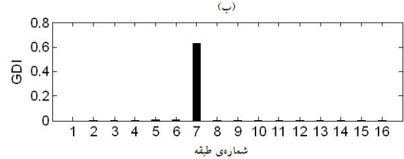
شکل ۲- نتیجه‌های مربوط به الگوی آسیب شماره (۱) در قاب برشی ۱۶ طبقه (الف) ضریب‌های وابستگی خاکستری، (ب) شاخص GDI
