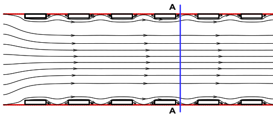
شکل ۱۲- خطوط جریان در میکروکانال برای z = 2w و w = 0.25H ، e = 5\% ، Re = 1 ، Kn = 0.0
