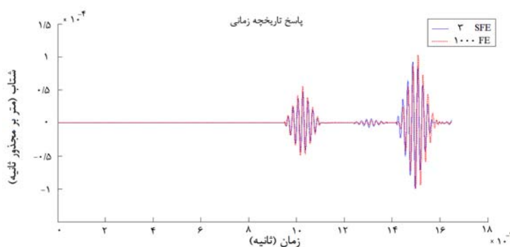
شکل ۷- شتاب طولی سر آزاد میله با جرم متمرکز ۰/۲ درصد جرم میله
