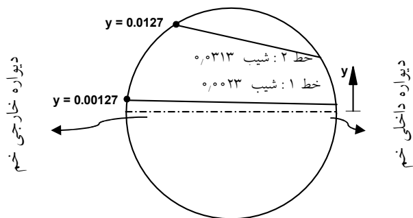
شکل ۴- موقعیت خطوط ۱ و ۲ (مشخص شده در شکل ۳) در یک مقطع اختیاری از لوله خمیده 180^\circ
