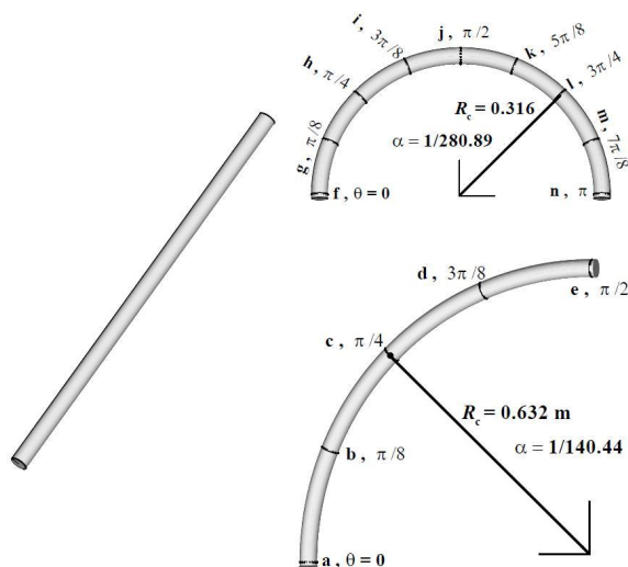
شکل ۱- هندسه‌های مورد بررسی
