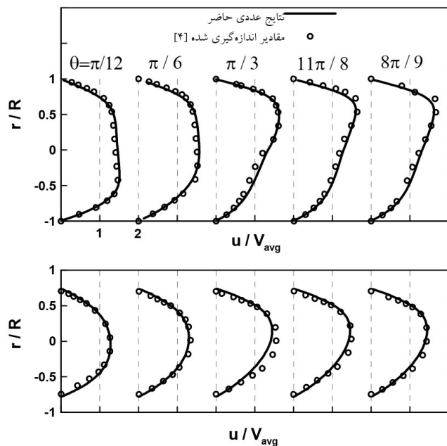
شکل ۳- سرعت بی بعد محوری در مقاطع مختلف خم 180^\circ در مقایسه با مقادیر اندازه گیری شده موجود در عدد رینولدز 242 ، (الف) روی خط ۱ و (ب) روی خط ۲ (مشخص شده در شکل ۴)
