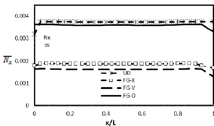
شکل ۲۰- منته تنش بی بعد در امتداد طول پوسته تکیه گاه ساده با V_{CN}^* = 0.17
