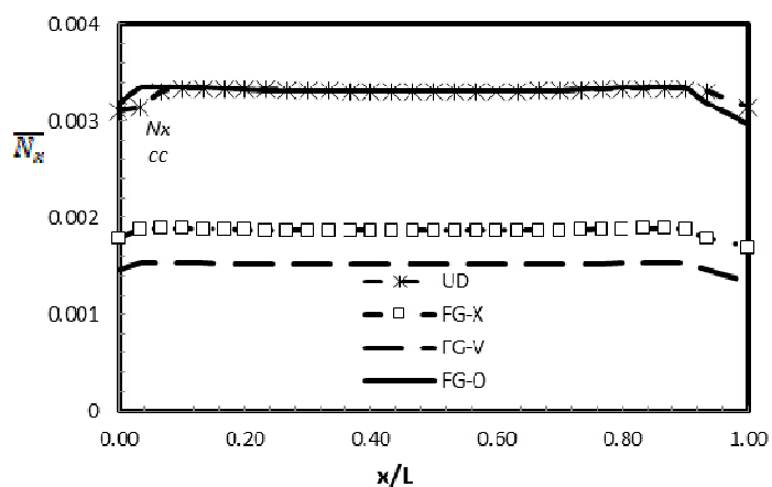
شکل ۱۹- منته تنش بی بعد در امتداد طول پوسته تکیه گاه گیردار با V_{CN}^* = 0.17
