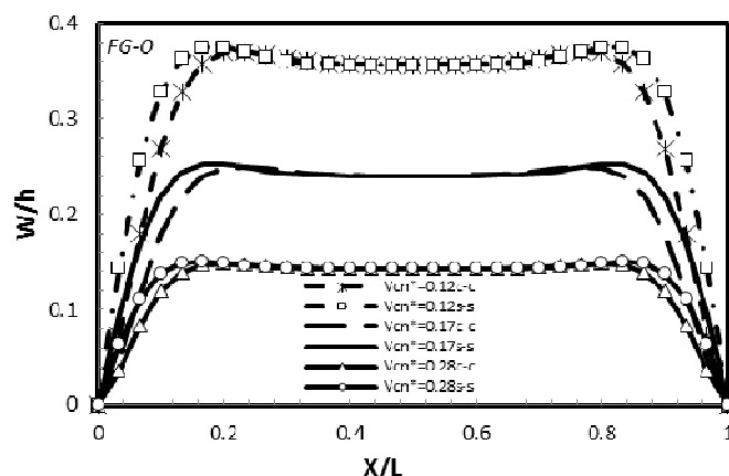
شکل ۱۸- تغییر خیز برحسب طول برای چیدمان FG-O و کسر حجمی مختلف نانولوله‌ها
