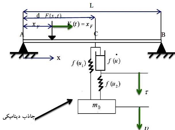
شکل ۱- تیر به همراه جاذب سه-المانه
