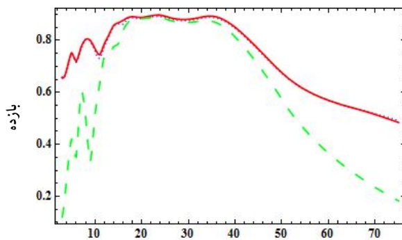
شکل ۱۷- نمودار بازده برحسب سرعت بار در حال حرکت (متر بر ثانیه)
