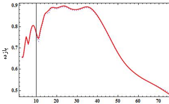
شکل ۱۵- نمودار بازده برحسب سرعت بار در حال حرکت؛ نقطه‌ها معرف جاذب دینامیکی دو- المانته خطی و خط پیوسته معرف جاذب دینامیکی سه- المانته خطی
