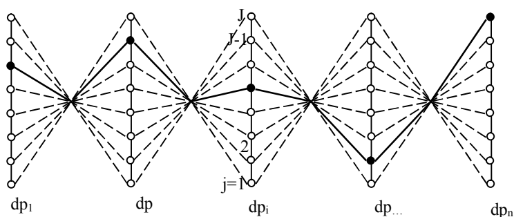
شکل ۲- گراف تعریف شده برای حل مسئله با استفاده از الگوریتم بهینه‌سازی جامعه مورچگان
