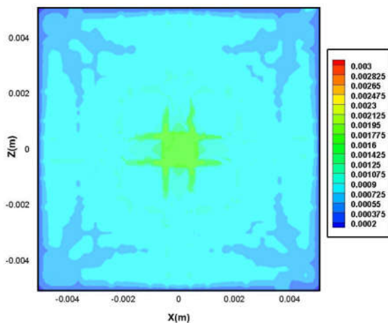
شکل ۶- توزیع کسر حجمی نانوذرات اکسید مس در در انتهای کانال (y = ۵۰ cm) در کسر حجمی متوسط \phi = ۰/۱\% و
