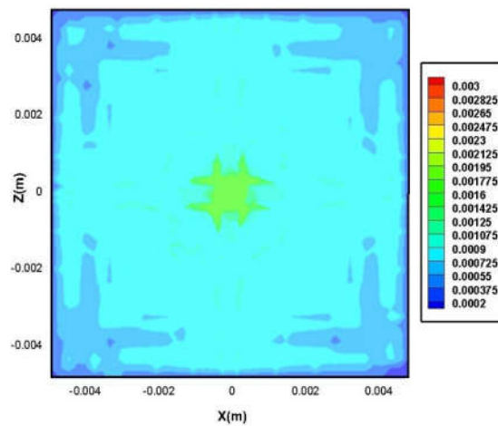
شکل ۵- توزیع کسر حجمی نانوذرات اکسید مس در انتهای کانال (y = ۵۰ cm) در کسر حجمی متوسط \phi = ۰/۱\% و
