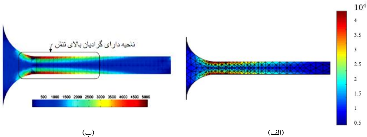
شکل ۱۳- مقایسه نتایج مربوط به توزیع تنش ون-مایسز
