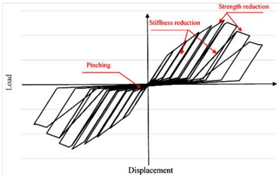
شکل ۱- ویژگی‌های منحنی رفت و برگشتی پنل گچی
