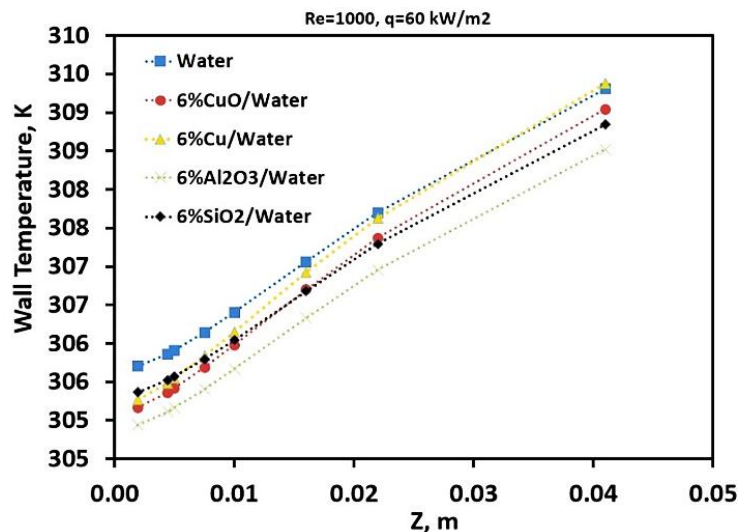
شکل ۷- تأثیر نوع نانوذره بر روی دمای دیواره با غلظت‌های یکسان
