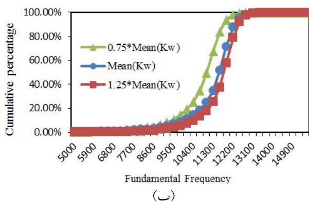
شکل ۱۳- نمودارهای: (الف) توزیع فراوانی و (ب) توزیع تجمعی، برای بسامدهای مود اول پیش‌بینی شده با استفاده از مدل جایگزین کریجینگ برای مقادیر \mu_{K_w} \times 0.75 ، \mu_{K_w} ، \mu_{K_w} \times 1.25 از پارامتر سفتی برشی ( K_w ).
