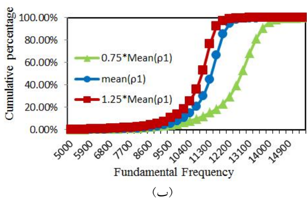
شکل ۱۴- نمودارهای: (الف) توزیع فراوانی و (ب) توزیع تجمعی، برای بسامدهای مود اول پیش‌بینی شده با استفاده از مدل جایگزین کریجینگ برای مقادیر \mu_{p_1} \times 0.75 ، \mu_{p_1} ، \mu_{p_1} \times 1.25 از پارامتر چگالی لایه اول ( p_1 ).
