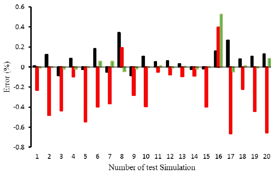
شکل ۶- خطای پاسخ‌های پیش‌بینی شده با استفاده از روش‌های Kriging، RBF و PRSM نسبت به روش حل سه‌بعدی برای بیست شبیه‌سازی تصادفی.
