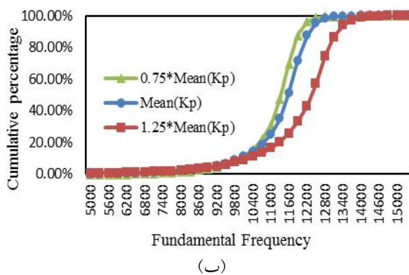
شکل ۱۲- نمودارهای: (الف) توزیع فراوانی و (ب) توزیع تجمعی، برای بسامدهای مود اول پیش‌بینی شده با استفاده از مدل جایگزین کریجینگ برای مقادیر \mu_{K_p} \times 0.75 ، \mu_{K_p} ، \mu_{K_p} \times 1.25 از پارامتر سفتی برشی ( K_p ).
