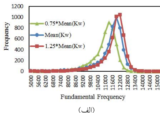
شکل ۱۳- نمودارهای: (الف) توزیع فراوانی و (ب) توزیع تجمعی، برای بسامدهای مود اول پیش‌بینی شده با استفاده از مدل جایگزین کریجینگ برای مقادیر \mu_{K_w} \times 0.75 ، \mu_{K_w} ، \mu_{K_w} \times 1.25 از پارامتر سفتی برشی ( K_w ).
