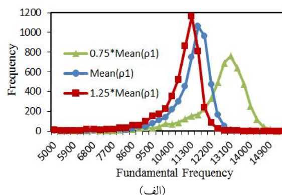
شکل ۱۴- نمودارهای: (الف) توزیع فراوانی و (ب) توزیع تجمعی، برای بسامدهای مود اول پیش‌بینی شده با استفاده از مدل جایگزین کریجینگ برای مقادیر \mu_{p_1} \times 0.75 ، \mu_{p_1} ، \mu_{p_1} \times 1.25 از پارامتر چگالی لایه اول ( p_1 ).
