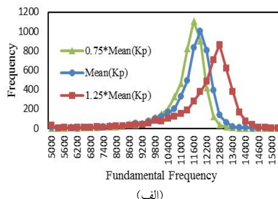
شکل ۱۲- نمودارهای: (الف) توزیع فراوانی و (ب) توزیع تجمعی، برای بسامدهای مود اول پیش‌بینی شده با استفاده از مدل جایگزین کریجینگ برای مقادیر \mu_{K_p} \times 0.75 ، \mu_{K_p} ، \mu_{K_p} \times 1.25 از پارامتر سفتی برشی ( K_p ).
