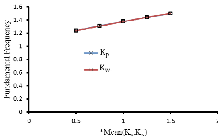
شکل ۹- نمودار تغییرات بسامد طبیعی مود اول ورق سه لایه مدرج FGMEE به ازای تغییرات مؤلفه‌های سفتی بستر ارتجاعی ( K_w, K_p ) حول مقدار میانگین متغیرها با استفاده از روش حل سه بعدی.
