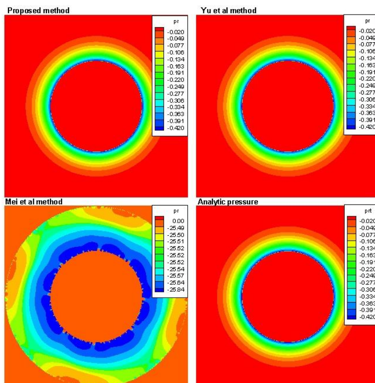
شکل ۱۱- مقایسه اندازه فشار بین دو استوانه برای معادله تحلیلی و شبیه‌سازی‌های انجام شده (رنگی در نسخه الکترونیکی)
