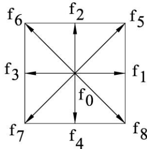
شکل ۱- یک مدل دوبعدی، شبکه ۹ سرعتی ( D_2Q_9 )
