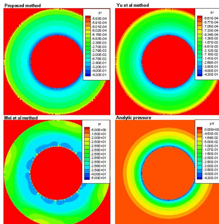
شکل ۱۲- مقایسه اندازه فشار برای معادله تحلیلی و شبیه‌سازی‌های انجام شده، نزدیک سطح استوانه داخلی و بیرونی (رنگی در نسخه الکترونیکی)
