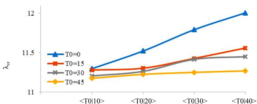
شکل ۸- ضریب بار کمانشی ورق کامپوزیت تک‌لایه با سختی متغیر با T_1 و T_0 مختلف با شرایط مرزی SSSS، \lambda_{cr} = \frac{\sigma_{cr} b^2}{E_y h^3}
