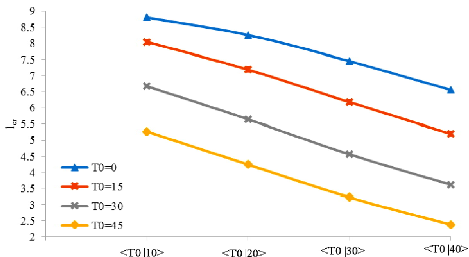
شکل ۹- ضریب بار کمانشی ورق کامپوزیت تک لایه با سختی متغیر با T_0 و T_1 مختلف با شرایط مرزی SFSF، \lambda_{cr} = \frac{\sigma_{cr} b^2}{E_v h^2}
