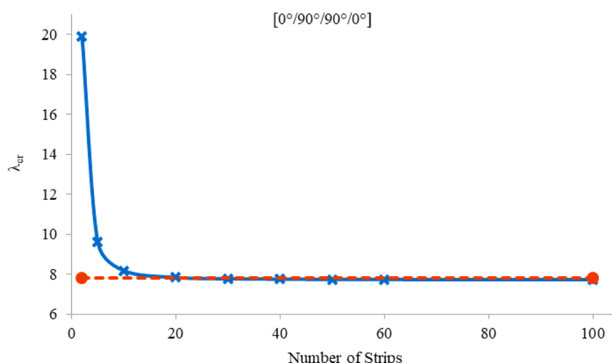
شکل ۷- تأثیر افزایش تعداد نوار بر ضریب بار کمانشی ورق کامپوزیت لایه‌ای با الیاف متعامد با شرایط مرزی SSSC
