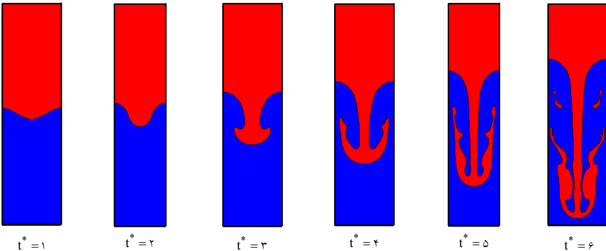
Re = 1024 (ب)
