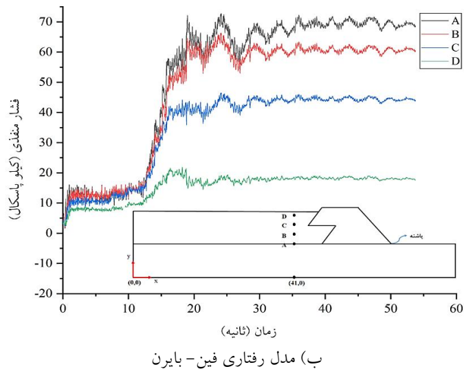
شکل ۸- فشار منفذی به دست آمده از دو مدل رفتاری موهر-کلمب و فین-بایرن در فاصله ۲۹ متری از پاشنه
