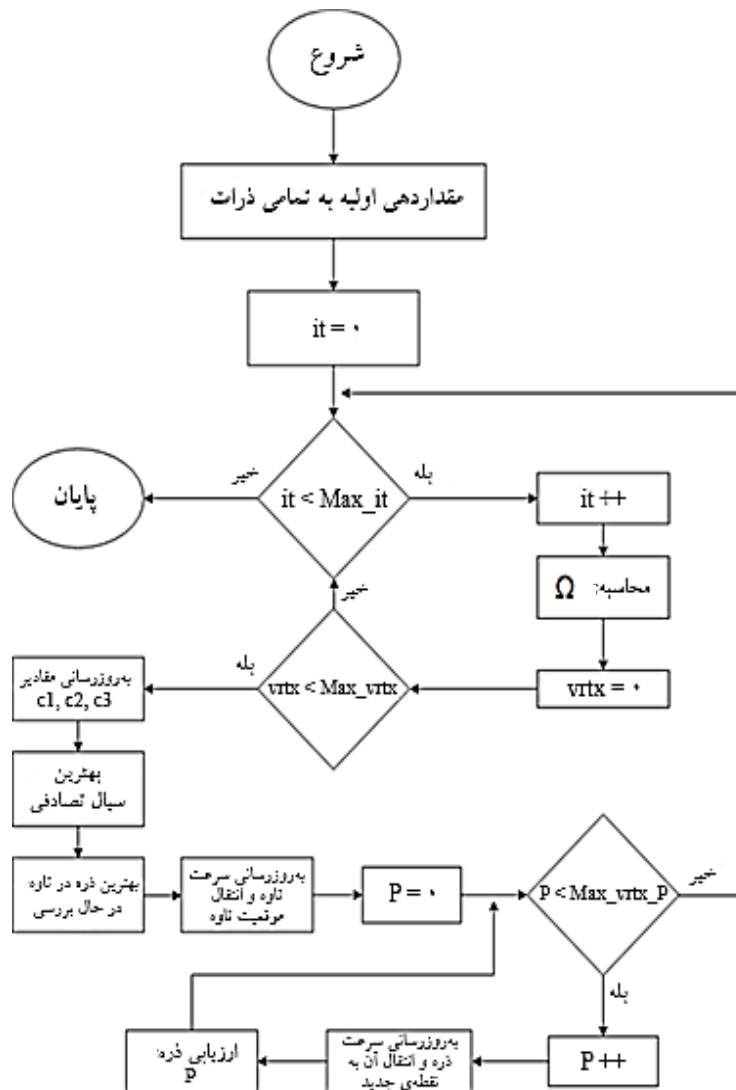
شکل ۶- فلوچارت روش فراابتکاری تاوه پیشنهادی
