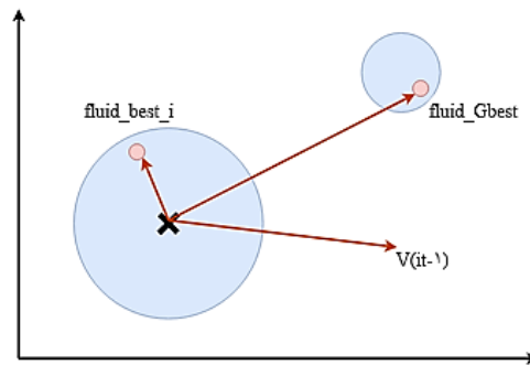
شکل ۳- بردارهای مورد استفاده در حرکت تاوه‌ها
