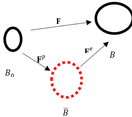
شکل ۱- تجزیه ضربی تانسور گرادیان تغییر شکل
