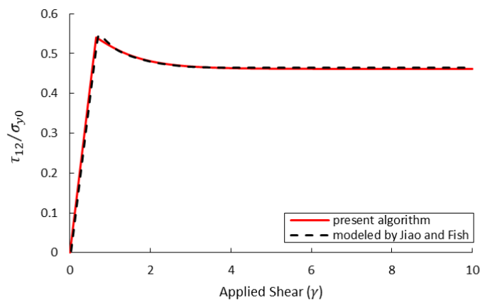
شکل ۷- نسبت \frac{\tau_{12}}{\sigma_{y0}} برای ماده‌ی جدول ۲ با در نظر گرفتن پلاستیسته کامل
