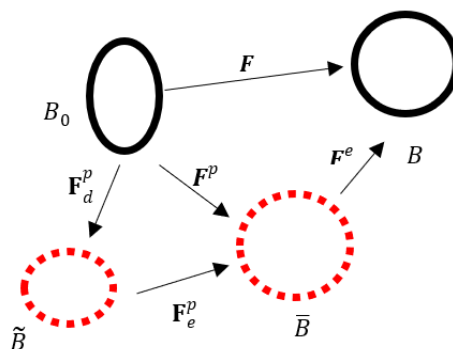
شکل ۲- تجزیه ضربی تانسور گرادیان تغییر شکل پلاستیک
