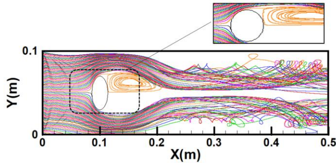
شکل ۲۰- خطوط مسیر ذرات برای ۱۰۰ ذره ۱۰ میکرومتری در Re=800 و F=1/44
