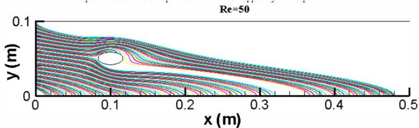
شکل ۸- درصد رسوب ذرات برای مانع در عدد رینولدز ۵۰ و نسبت اقطار ۰/۵ برای ۱۰۰ ذره ی ۱۰ میکرونی ۶ درصد است [۳۰].
