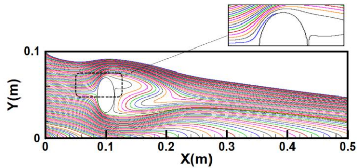
شکل ۱۸- خطوط مسیر ذرات برای ۱۰۰ ذره‌ی ۱۰ میکرومتری در Re=200 و F=1/44
