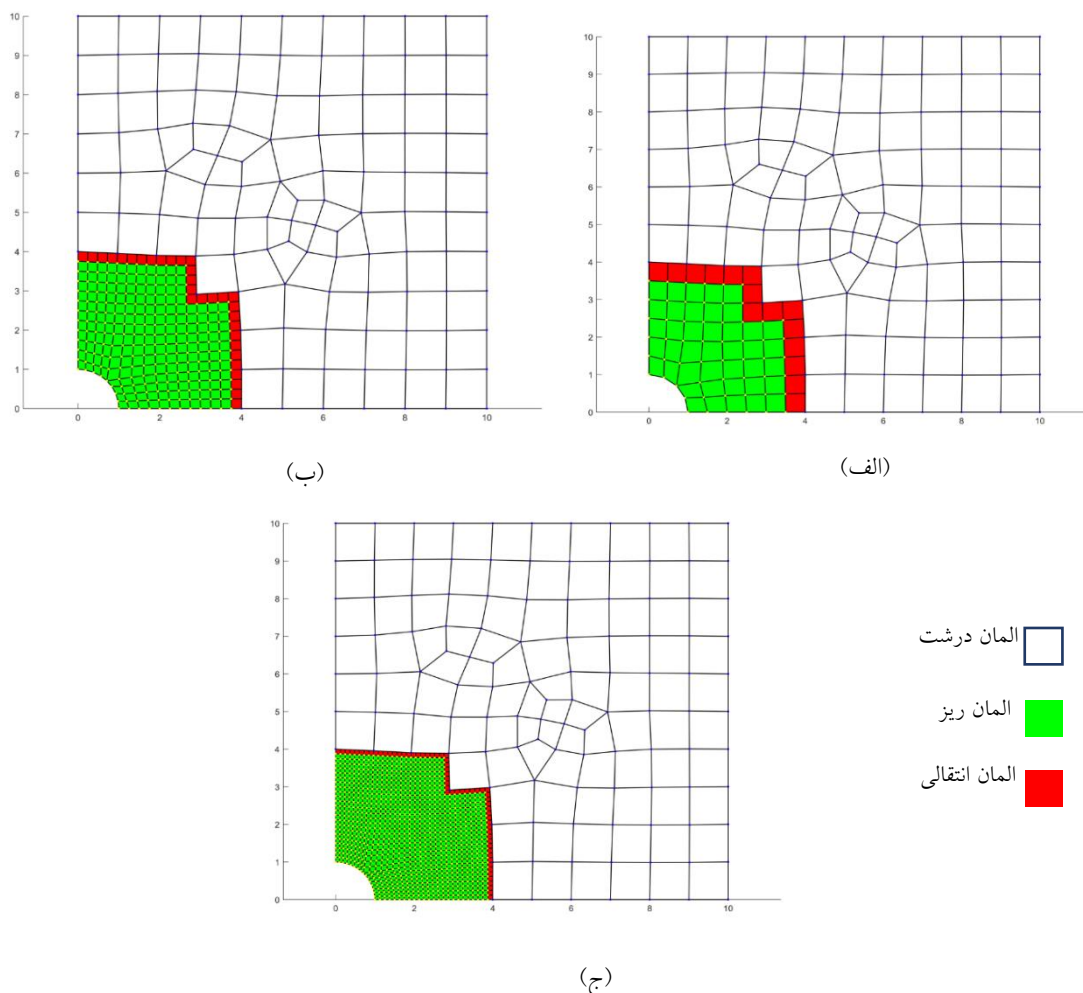
شکل ۱۹- شبکه‌بندی‌های متفاوت در حالت شبکه ریزشده با نسبت‌های دلخواه بر اساس روش توابع شکل پیشنهادی: الف) ۵/۰ - ۱ میلی‌متر، ب) ۲۵/۰ - ۵/۰ میلی‌متر، ج) ۱۲۵/۰ - ۲۵/۰ میلی‌متر
