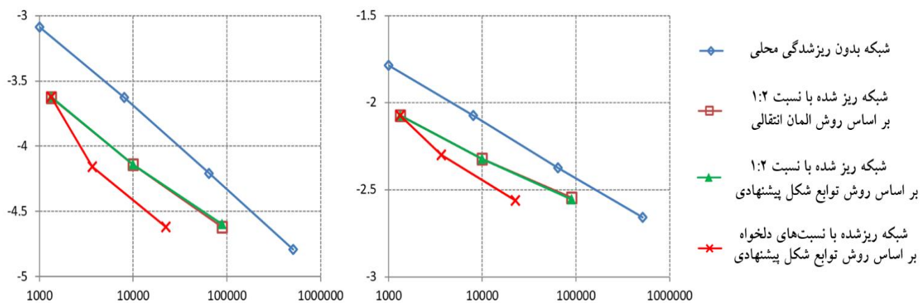
شکل ۲۴- نمودارهای همگرایی بر حسب تعداد المان‌های شبکه برای مثال مکعب دارای حفره کروی شکل: الف) نرم خطای جابجایی ب) نرم
