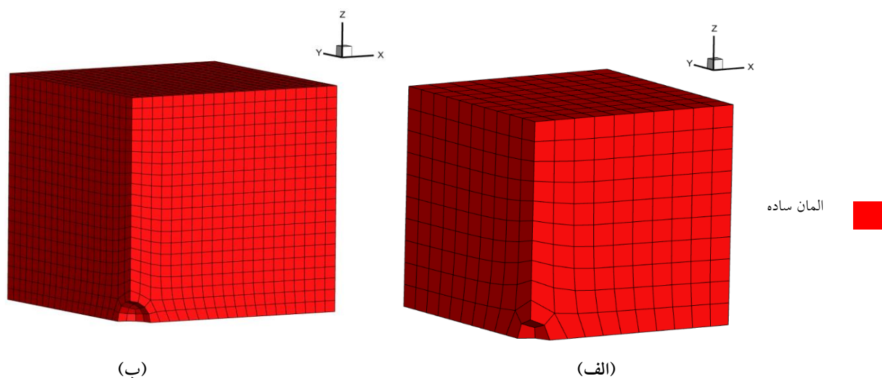
شکل ۲۱- شبکه بندی های متفاوت در حالت شبکه بدون ریز شدگی محلی با اندازه المان‌های: الف) ۱ میلی‌متر، ب) ۰/۵ میلی‌متر
