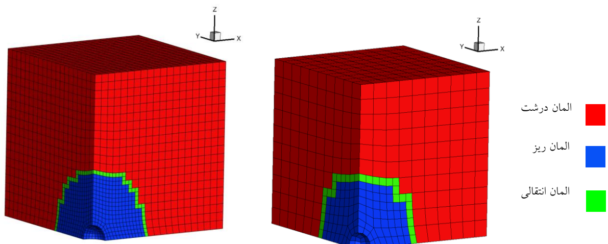
شکل ۲۳- شبکه بندی های متفاوت در حالت شبکه ریز شده با نسبت ۱:۲ بر اساس روش توابع شکل پیشنهادی با اندازه المان‌های: الف) ۰/۵ -
