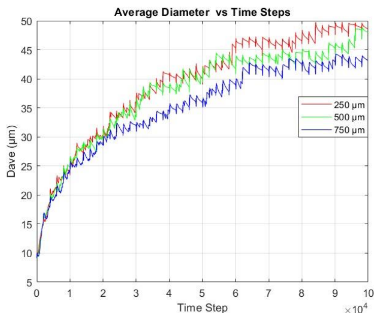
شکل ۹. نمودار اندازه متوسط دانه بر حسب زمان برای حجمک نماینده در عمق‌های ۲۵۰، ۵۰۰ و ۷۵۰ میکرومتر
