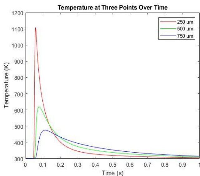
شکل ۸. تغییرات دما در طول زمان برای سه نقطه در عمق‌های ۲۵۰، ۵۰۰ و ۷۵۰ میکرومتر
