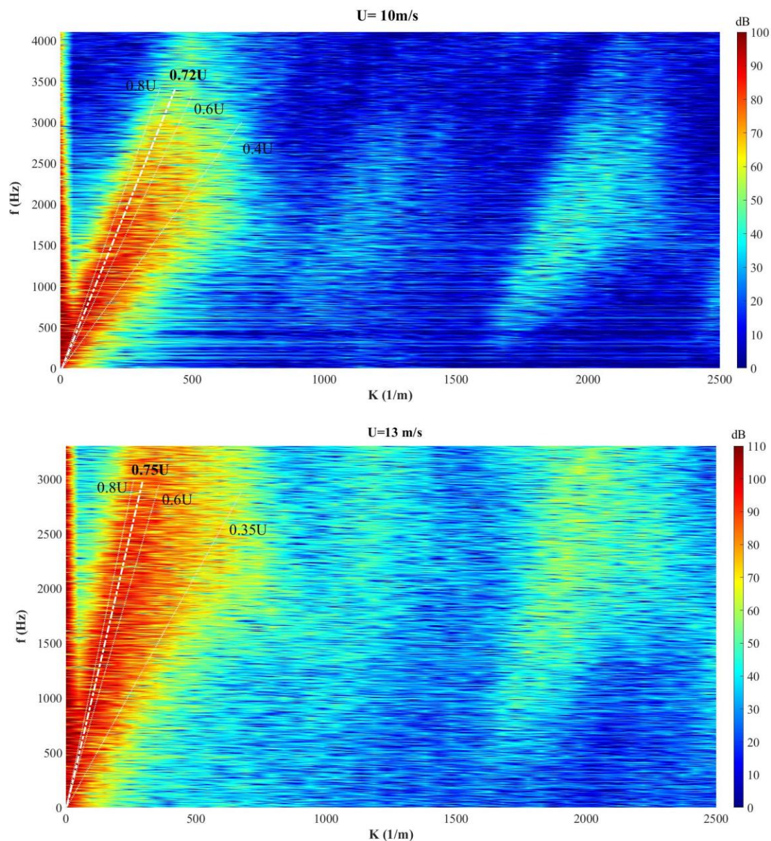
شکل ۱۱. تغییرات فشار لحظه‌ای ثبت شده بر دیوار در فضای فرکانس-عدد موج در سرعت‌های مختلف جریان. نوار قرمز رنگ نشان دهنده برجستگی همرفتی است که برای محاسبه سرعت متوسط جابجایی ساختارهای آشفتگی در مجرا بکار می‌رود.
