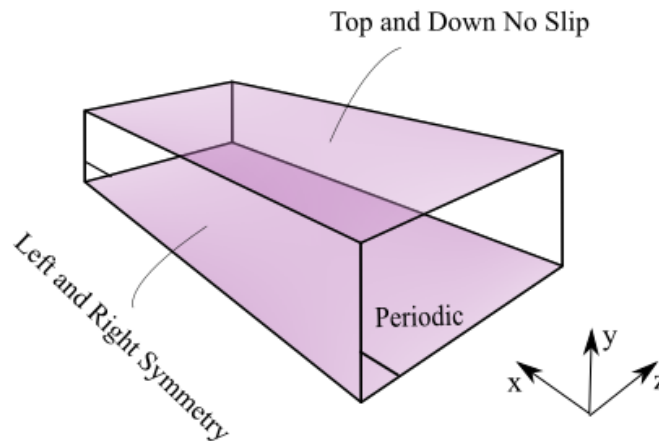
شکل ۱ طرح‌واره جریان تناوبی داخل کانال
