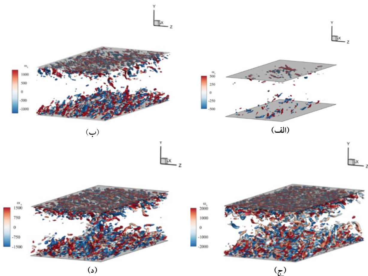
شکل ۷. سطوح هم‌تراز معیار Q و کانتور چرخش (ورتیسیته) در سرعت‌های مختلف: (الف) ۵/۵ متر بر ثانیه، (ب) ۸ متر بر ثانیه، (ج) ۱۰ متر بر ثانیه، (د) ۱۳ متر بر ثانیه.
