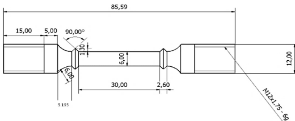
شکل ۱. هندسه نمونه در استاندارد ASTM E139-11 آزمون تنش گسیختگی [۱۶].
