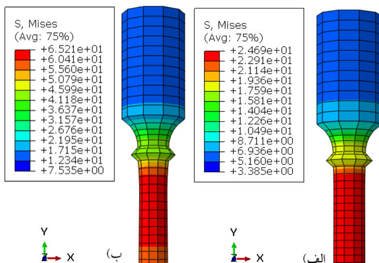
شکل ۷. کانتوهای توزیع تنش در زمان پایانی با مدل های الف) قانون توان و ب) تتا پروجکشن.
