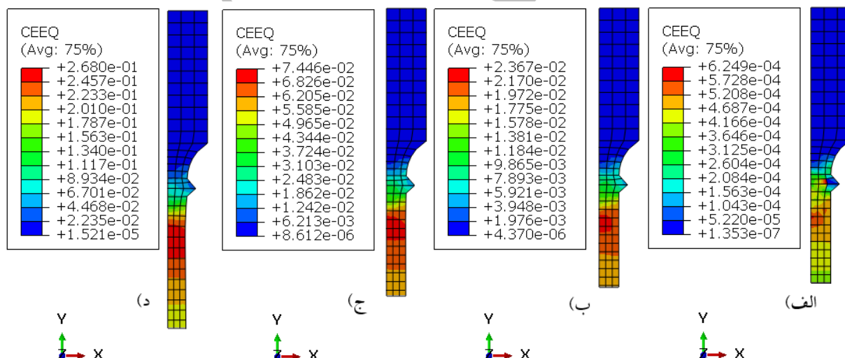
شکل ۶. توزیع خطوط CEEQ در دمای ۹۵° درجه سلسیوس و تنش ۲۲ مگاپاسکال با مدل تتا پروجکشن در الف) ثانیه های اولیه، ب) ۱۰۰ ساعت، ج) ۲۲۰ ساعت و د) زمان پایانی.
