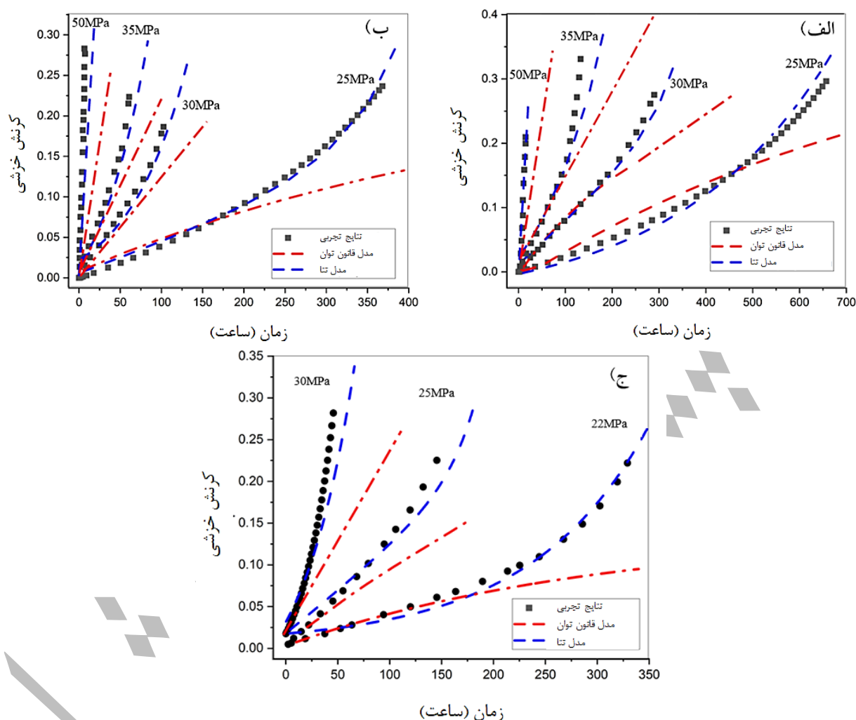
شکل ۳. مقایسه کرنش خزش با دو مدل قانون توان و تتا پروجکشن با نتایج تجربی در دماهای الف (۹۰۰، ب) ۹۲۵ و ج) ۹۵۰ سلسیوس در تنش های مختلف.
