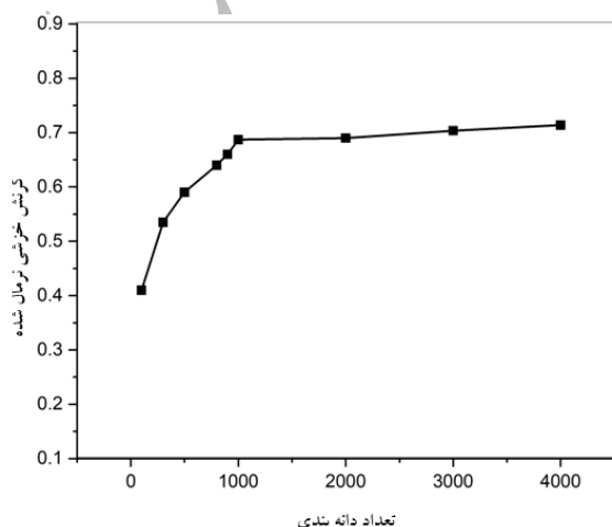
شکل ۴. تاثیر تعداد المانها در الف) کرنش خزشی نرمال شده و ب) تنش های فون میزز
