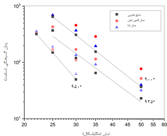
شکل ۴. نمودار لگاریتم مقایسه زمان گسیختگی برحسب لگاریتم تنش در مدل های خزشی قانون توان و تننا پروجکشن.
