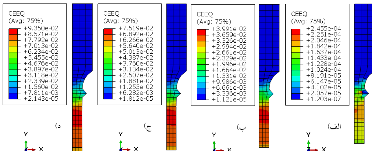
شکل ۵. توزیع خطوط CEEQ در دمای ۹۵° درجه سلسیوس و تنش ۲۲ مگاپاسکال با مدل قانون توان در الف) ثانیه های اولیه، ب) ۱۰۰ ساعت، ج) ۲۲۰ ساعت و د) زمان پایانی.
