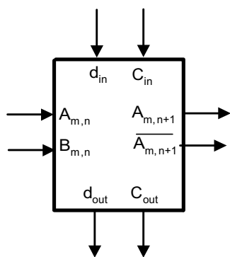
شکل ۲ - عنصر پردازشی اصلی ساختمان آرایه سیستولیک
