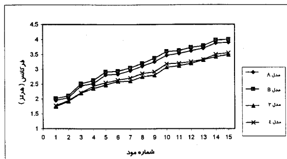
شکل ۶- تأثیر نحوه اعمال مشخصات مصالح بر فرکانسهای طبیعی ۱۵ مود اول ارتعاشی سد مارون
