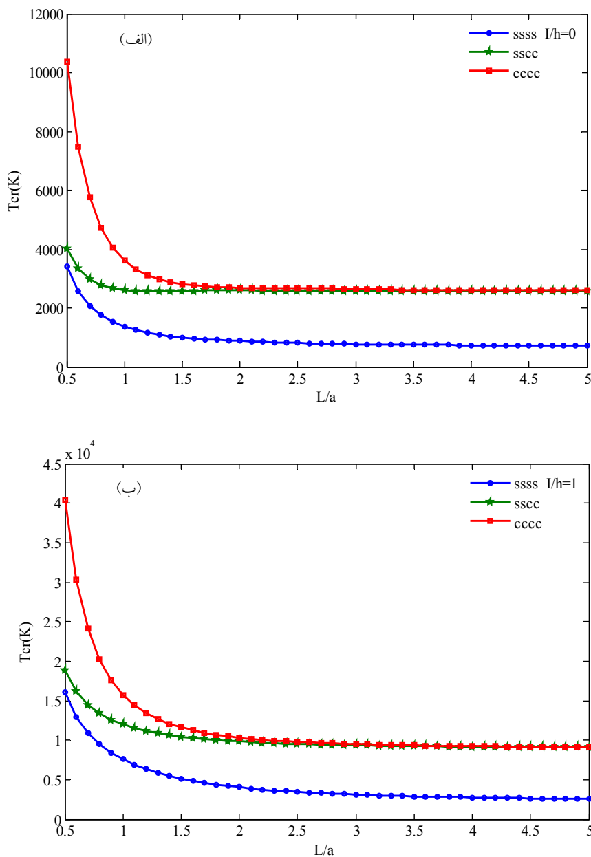
شکل ۲- تغییرات دمای بحرانی کمانش ورق برحسب نسبت طول به عرض در حالت توزیع یکنواخت دما
