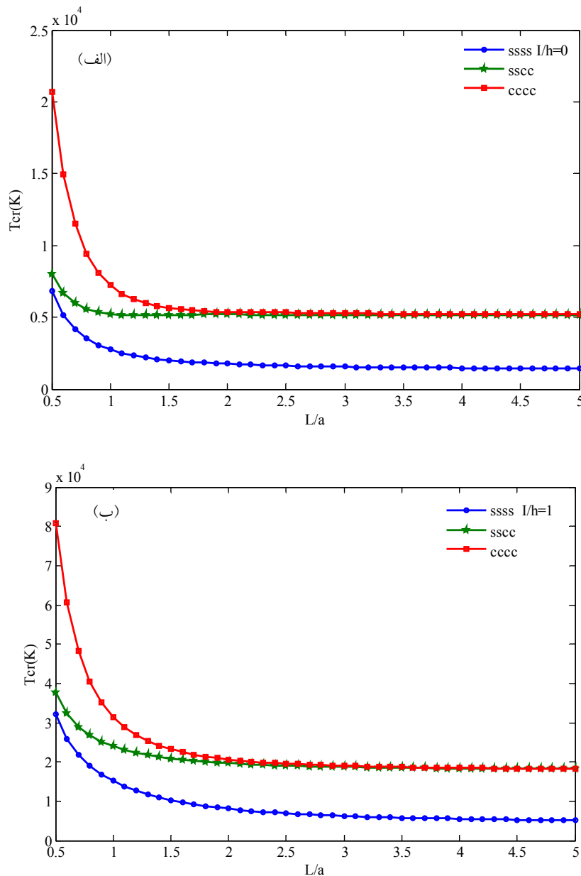
شکل ۳- تغییرات دمای بحرانی کمانش ورق بر حسب نسبت طول به عرض در حالت توزیع خطی دما
