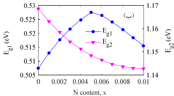
شکل ۳- الف) اتلاف گرمایی و ب) مقادیر زیرگاف‌های انرژی E_{g1} و E_{g2} مربوط به \text{InAs}_{(1-x)}\text{N}_x/\text{AIP}_{0.7}\text{Sb}_{0.3} QD-IBSC برحسب غلظت مولی نیتروژن، x
